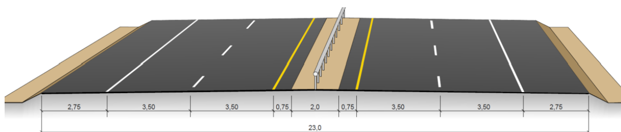
Figur 2-1. Tverrprofil for H3. H3 kan ha en veibredde på 21 - 23 m og midtdeler med rekkverk. Kilde: Håndbok N100 Veg- og gateutforming, Statens vegvesen (Statens vegvesen, 2019)
