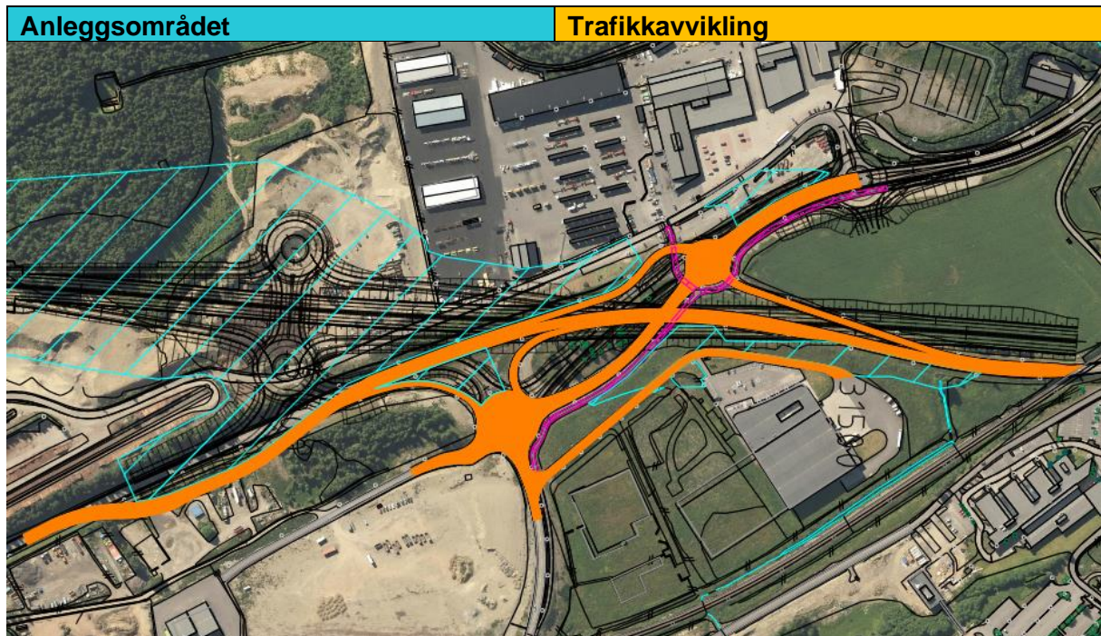
Figur 2-40 Utklipp fra prinsippskisse TEGN-vei-999_Y3203 og Y3303
