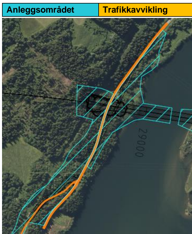
Figur 2-26 Utklipp fra prinsippskisse TEGN-vei-999_Y3103
