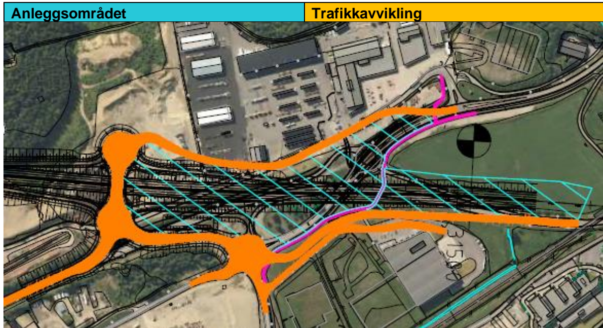
Figur 46 Utklipp fra prinsippkisse TEGN-vei-999_Y3503
