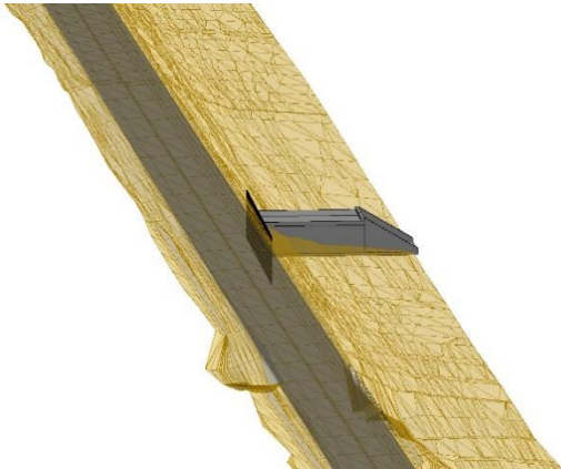
Figur 1-2 Generell illustrasjon over utførelse kulvert Fase 1
