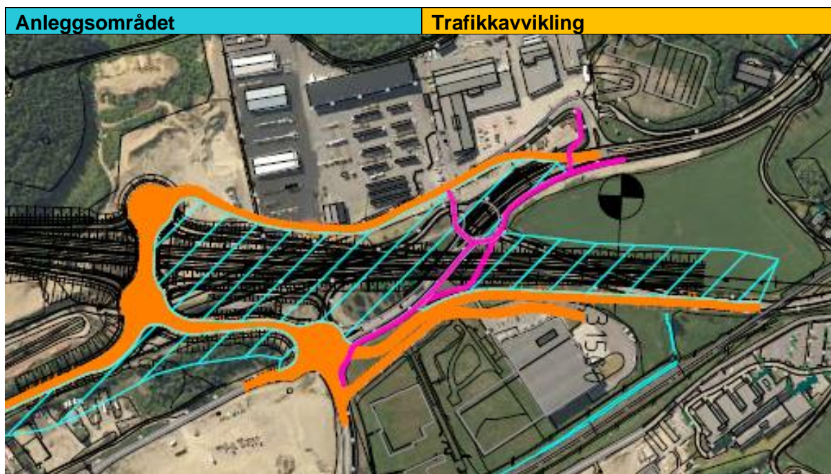
Figur 2-41 Utklipp fra prinsippskisse TEGN-vei-999_Y3403
