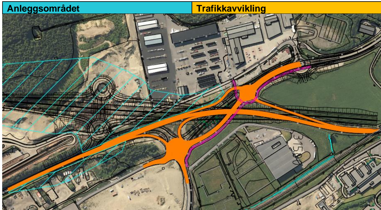
Figur 2-39 Utklipp fra prinsippskisse TEGN-vei-999_Y3103
