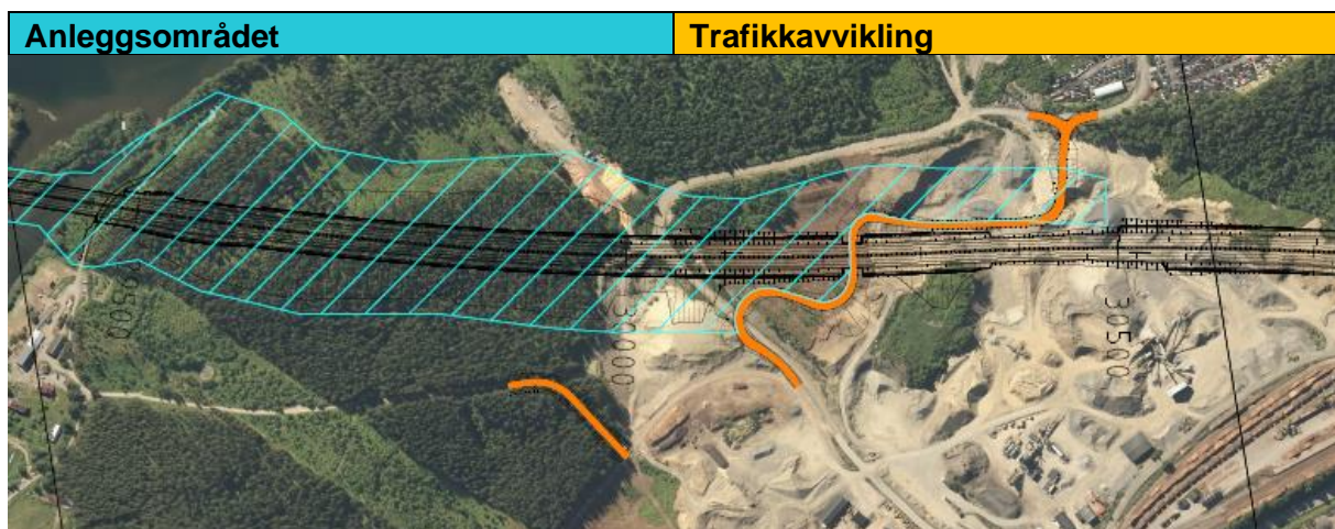
Figur 2-36 Utklipp fra prinsippskisse TEGN-vei-999_Y3203
