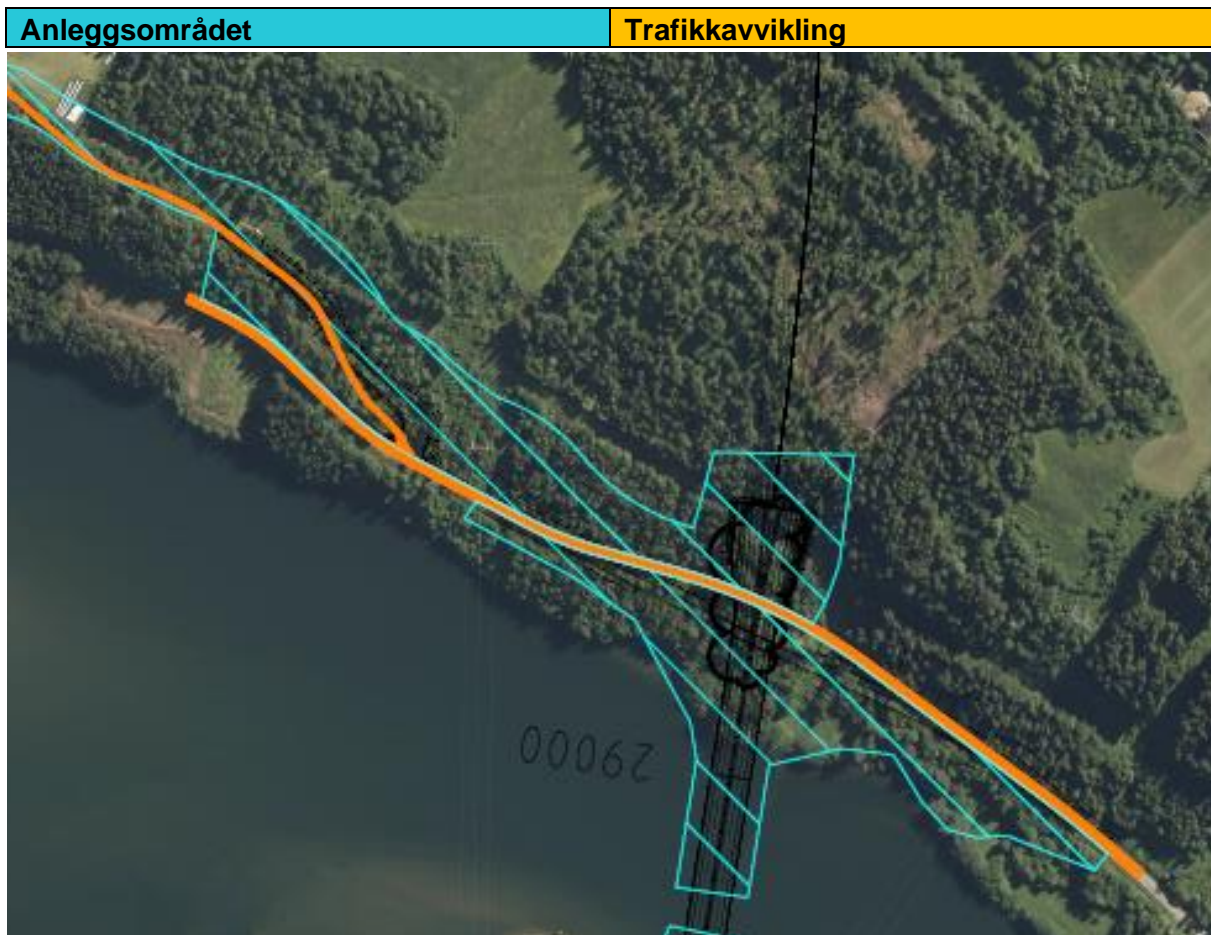
Figur 2-25 Illustrasjonsbilde av påhuggsområdet hentet fra faseplaner, prinsippskisse TEGN-vei-999
