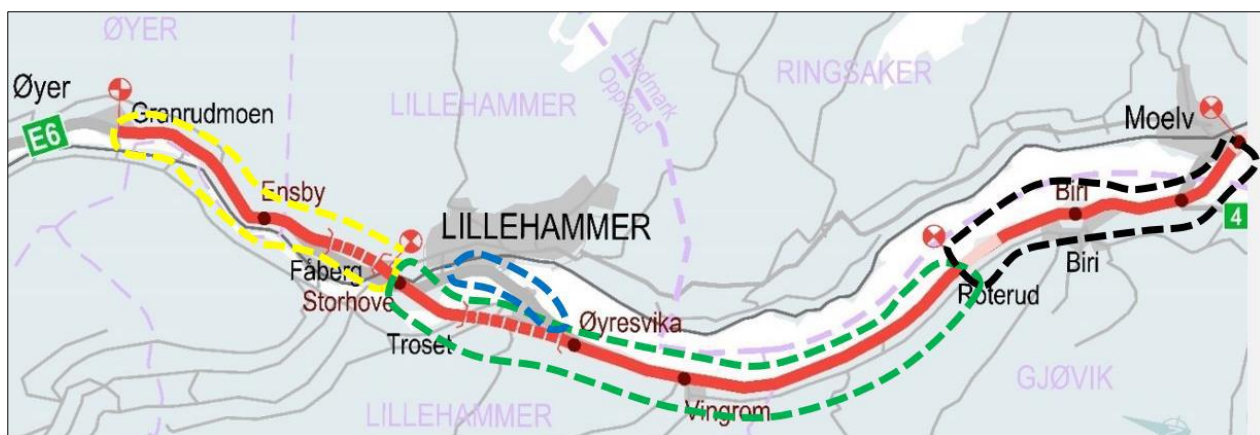
Figur 1. Oversiktsskisse over E6 Moelv-Øyer. E6 Roterud Storhove, er vist med grønn stiplet linje.
