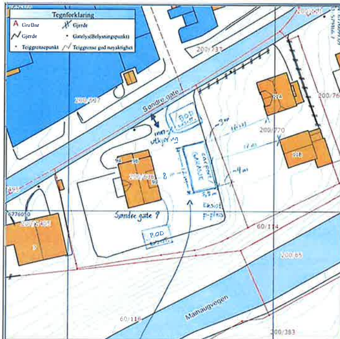
Situasjonskart med inntegnet plassering av planlagt garasje
